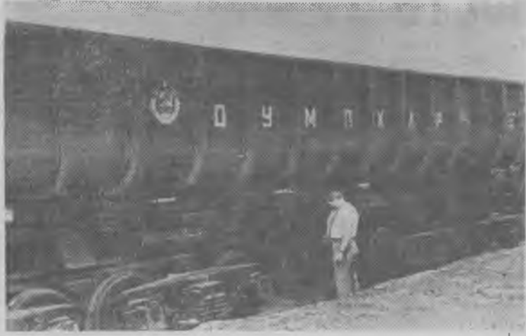
ДНЕПРОДЗЕРЖИНСК. Конструкторы вагоностроительного завода имени газеты «Правда» успешно работают над созданием новых, более совершенных саморазгружающихся вагонов для перевозки различных народнохозяйственных грузов. Закончились заводские испытания нового облегченного 120-тонного думпкара, приспособленного для перевозки руды. Этот цельнометаллический посылочный вагон-самосвал создан конструкторами завода под руководством П. А. Кочешкова. НА СНИМКЕ: новый 120-тонный думпкар.
