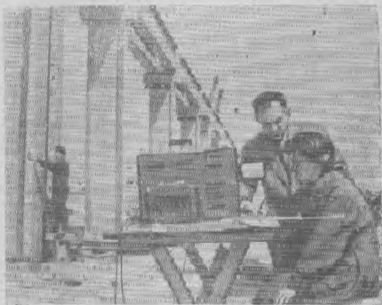
В научно-исследовательском институте строительства и архитектуры Украинской ССР создана оригинальная установка для испытаний бетона. Ее автор инженер С. И. Ногин. Это ультразвуковая сварочная «скорая техническая помощь». Шипы прибора передают в толщу бетона ультразвуковые волны, при помощи которых определяются прочность материала, его однородность, внутренние дефекты — растрескивание, трещины. Ультразвуковые измерения можно производить в конструкциях толщиной от 5 сантиметров до 10 метров.
