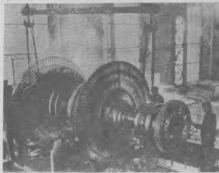
На Харбинском заводе турбогенераторов создана первая в стране паровая турбина мощностью 100 тысяч киловатт. НА СНИМКЕ: установка ротора турбины.
