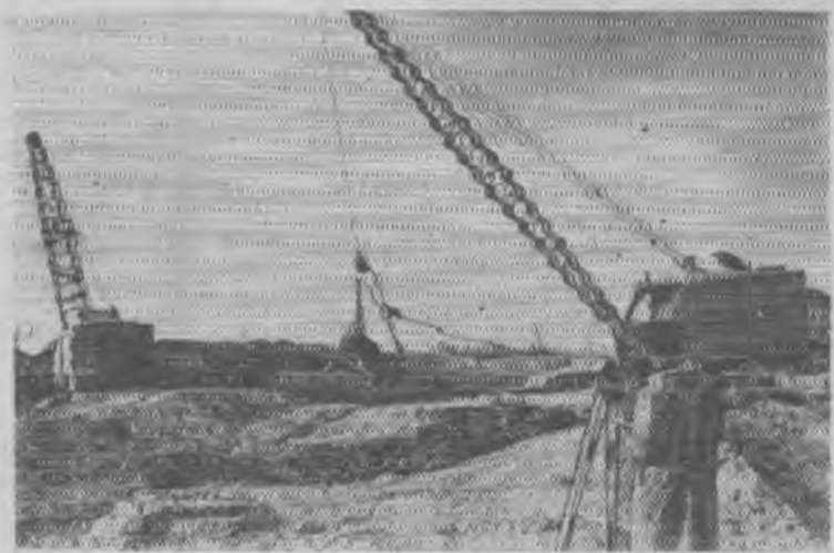
Казахская ССР. На юге республики в Голодной степи ведется строительство Южного Голодноостепского канала. Строители решили в ближайшие два-три года дополнительно освоить 21 тысячу гектаров новых земель. Они построили главное ответвление основной южной трассы протяженностью 20 километров, выбросив 1,5 миллиона кубометров грунта.
