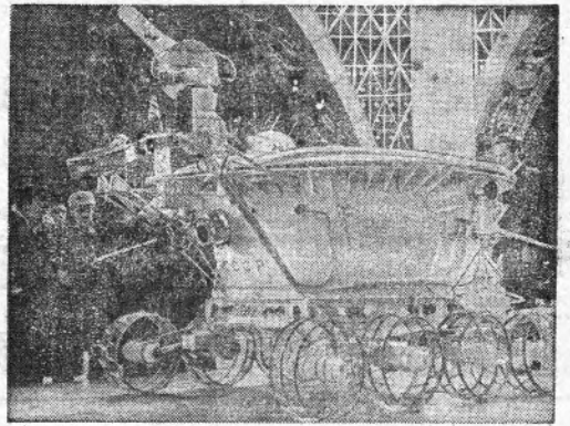
МОСКВА. Экспозиция павильона «Космос» Выставки достижений народного хозяйства СССР пополнилась новым уникальным экспонатом. Здесь установлена точная копия первой передвижной автоматической лаборатории «Луноход-1» для комплексного изучения особенностей строения лунной поверхности, окололунной среды и дальних космических объектов. Фото Н. Хренникова (Фотохроника ТАСС).
