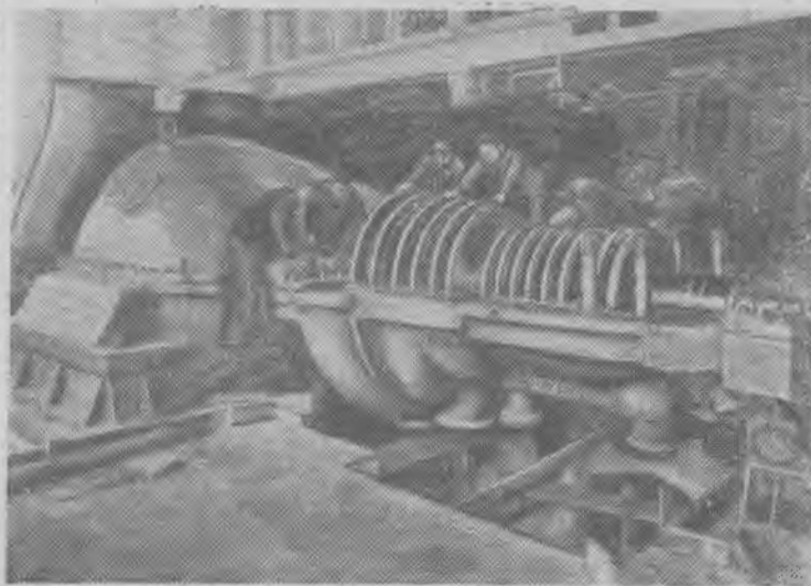
Венгерская Народная Республика. В ближайшее время энергетическое хозяйство республики пополнится новым промышленным объектом—теплоэлектростанцией Типапалконье. На снимке: монтаж турбины мощностью 50.000 киловатт.
