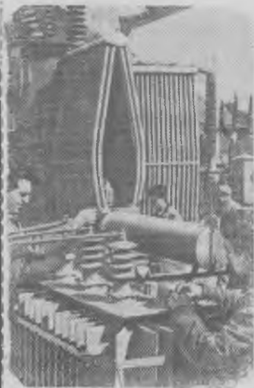
На Софийском заводе имени Василия Коларова. На снимке: электромонтажишники проверяют трансформатор, предназначенный для электростанции "Пасарел".
