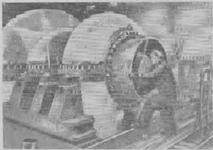
На Невском машиностроительном заводе имени В. И. Ленина изготавливается оборудование для газопровода Ставрополь—Москва—Ленинград. Осваивается производство газовых турбин мощностью 4.000 киловатт и нагнетателей газа, перекачивающих в одну минуту 280 кубометров газа под давлением в 55 атмосфер. Применение этого оборудования позволит пропускать газопровод и обеспечит бесперебойность его работы. Собрана и поставлена на испытание первая партия газовых турбин, идет сборка нагнетателей.
