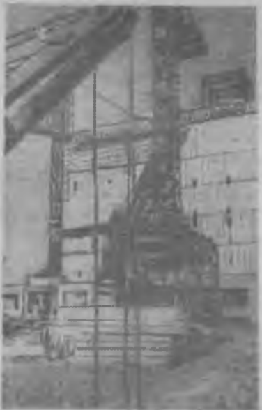
Свердловская область. Строители Белоярской атомной электростанции успешно справились с возведением здания реакторного отделения. Сейчас здесь ведутся отделочные работы.
