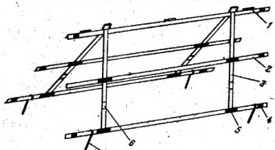
Малая теплица круглогодичного использования: 1 — шарнирное соединение, 2 — продольная рейка, 3 — боковая рейка, 4 — стыковочная пластина, 5 — зажим, 6 — соединение боковых реек, 7 — якорный штырь, 8 — крепеж
