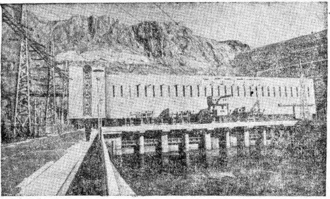
УЗБЕКСКАЯ ССР. Более 6 миллиардов киловатт-часов электроэнергии со дня пуска первого агрегата (декабрь 1970 года) вырабатала Чарвакская ГЭС. Станция полностью окупила расходы на свое строительство.
