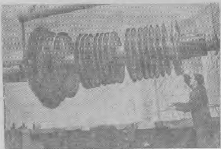
Калужский турбинный завод, выпускавший агрегаты мощностью до 12 тысяч киловатт, освоил выпуск машин мощностью 25 тысяч киловатт. В настоящее время здесь собирают турбину новой мощности.
