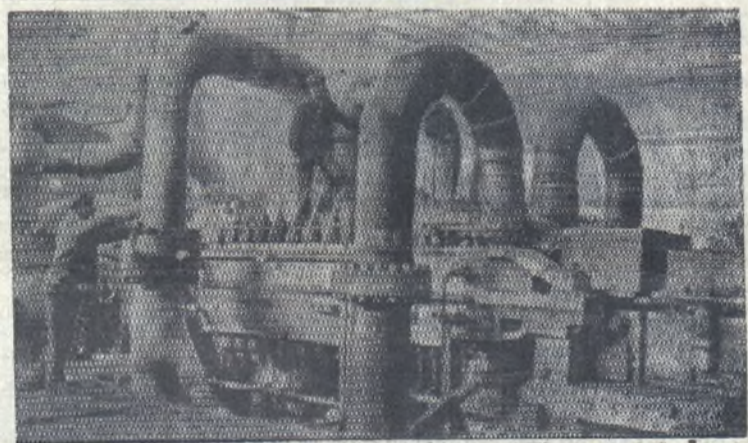
Крупнейшая в Сибири Назаровская ГРЭС — энергетический гигант, строящийся в Красноярском крае. К юбилею Октября здесь войдет в строй сверхмощный блок в полмиллиона киловатт (на снимке). Фото А. Татаренко.
