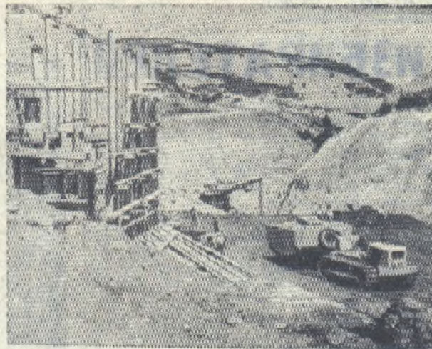
Алжир. На реке Арба в горах Большой Кабилии ведется строительство земляной плотины, которая позволит оросить свыше 600 гектаров засушливых земель. Это лишь одна из двадцати двух малых и средних плотин, которые будут возведены в Алжире по советским проектам. Советские специалисты оказывают техническое содействие в производстве работ и помогают готовить национальные кадры. Фото А. Богомаза. Фотохроника ТАСС.
