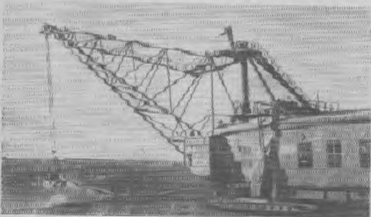
Механизаторы комбината «Узбекуголь» успешно применяли на открытых горных выработках в Ангренском угольном разрезе мощный шагающий экскаватор ЭШ 6-60. За тридцать суток во внутренние отвалы отгружено более 80 тысяч кубометров вскрышной породы.
