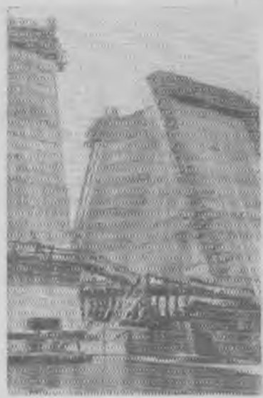
Строительство Флайской плотины в Чехословацкой Республике. Она будет состоять из 35 блоков. Ее высота достигнет 50 метров.
