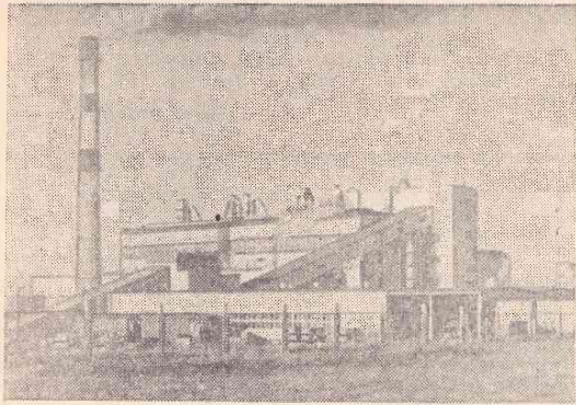
Монгольская Народная Республика. Общий вид Дарханской ТЭЦ, построенной с помощью Советского Союза. Фото В. Мاستюкова.
