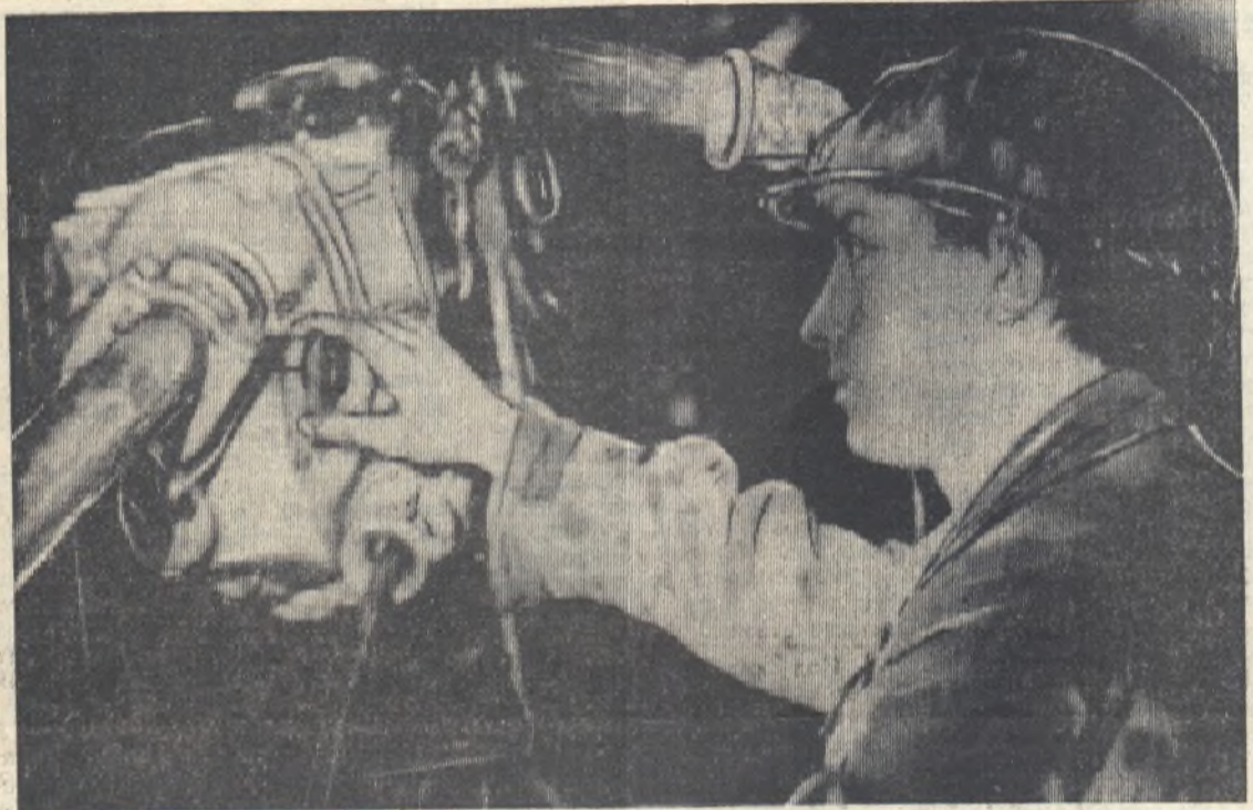
Добрая слава прошла по проходческим бригадам шахты Буланаш-25 о новой погрузочной машине ППМ-4М. Эта машина оборудована лопатой, которая достает породу в любом углу забоя. Кроме этого, на пневмостойках спереди машины устанавливаются для бурения шпуров 2 перфоратора, обладающих двухскоростной подачей и реверсом бура. НА СНИМКЕ: член бригады коммунистического труда, которой руководит В. Е. Семьяченко, проходчик Владимир Грудцын работает на новой машине при проходке западного квершлага горизонта 130 метров. Фото А. ГАЕВА.
