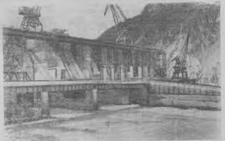
Восточно-Казахстанская область. Строители Бухтарминской ГЭС, соревнуясь в честь 42-й годовщины Великого Октября, одержали еще одну трудовую победу. Они перекрыли последний, третий по счету, пролет плотины. 250-тонный щит строительного затвора закрыл путь водам Иртыша, которые текут теперь только через донные отверстия двух первых пролетов.
