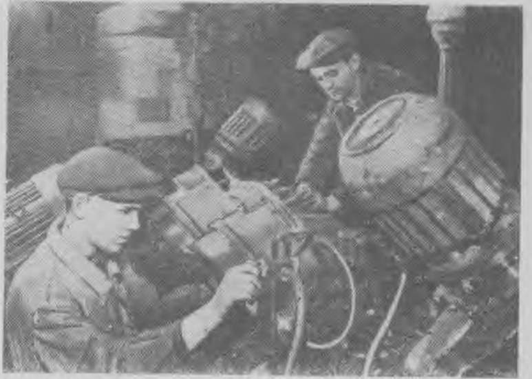
Москва. Осуществляя задачи семилетнего плана, работники научно-исследовательского института тракторного и сельскохозяйственного машиностроения создали первую в стране автоматическую линию для производства вкладышей режущих аппаратов сельскохозяйственных комбайнов. Она позволит изготовить до 26 миллионов вкладышей в год и полностью обеспечит потребность сельскохозяйственного машиностроения страны в этих деталях.
