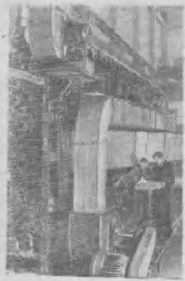
Иваново. На заводе текстильного машиностроения закончена сборка машины «АТО-110». Она предназначена для термической обработки хлопчатобумажных и штапельных тканей, предварительно пропитанных специальными химическими препаратами. Применение новой машины повышает качество тканей. Они приобретают свойства безусадочности, нестираемости и водоустойчивости. Производительность машины достигает 3,000 метров в час. Обслуживают ее два человека.
