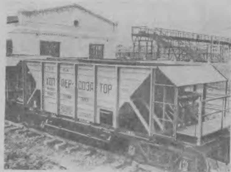
На Великолукском паровозостроительном заводе освоено производство хоппер-дозаторов специальных вагонов, предназначенных для строителей путейцев. Хоппер-дозатор позволяет автоматически, на ходу производить отсыпку щебня и балласта при сооружении или реконструкции железнодорожного пути. Пневматические механизмы полностью заменяют ручной труд на тяжелых строительных путевых работах.
