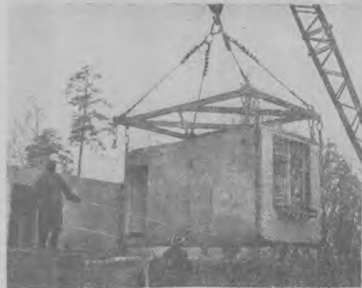
Строители треста № 104 «Главленинградстрой» начали монтаж первого в Ленинграде экспериментального восьмиквартирного дома из объемных элементов — блок-коробок, изготовленных и отлитых на заводе железобетонных изделий № 12. Такой метод строительства позволяет перенести большинство трудоемких операций в заводские условия. Это до минимума сокращает затраты труда на стройплощадке, значительно ускоряет строительство и удешевляет стоимость зданий.
