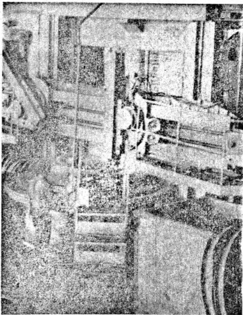
Крупные детали вентиляторов—кожуха, насадки, флянцы, рабочие колеса, звенья направляющих аппаратов и другие обрабатываются на металлорежущих станках, подобных этому—карусельному (на снимке слева).
